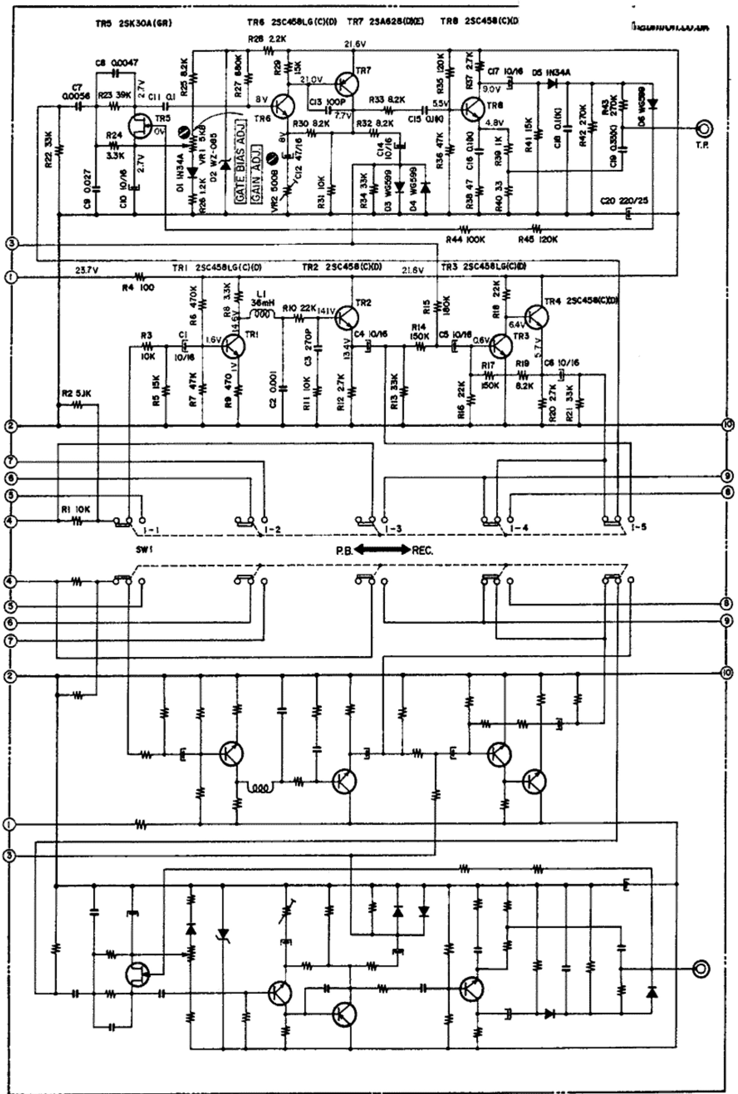
DOLBY N.R. P.C. BOARD LE-5037
